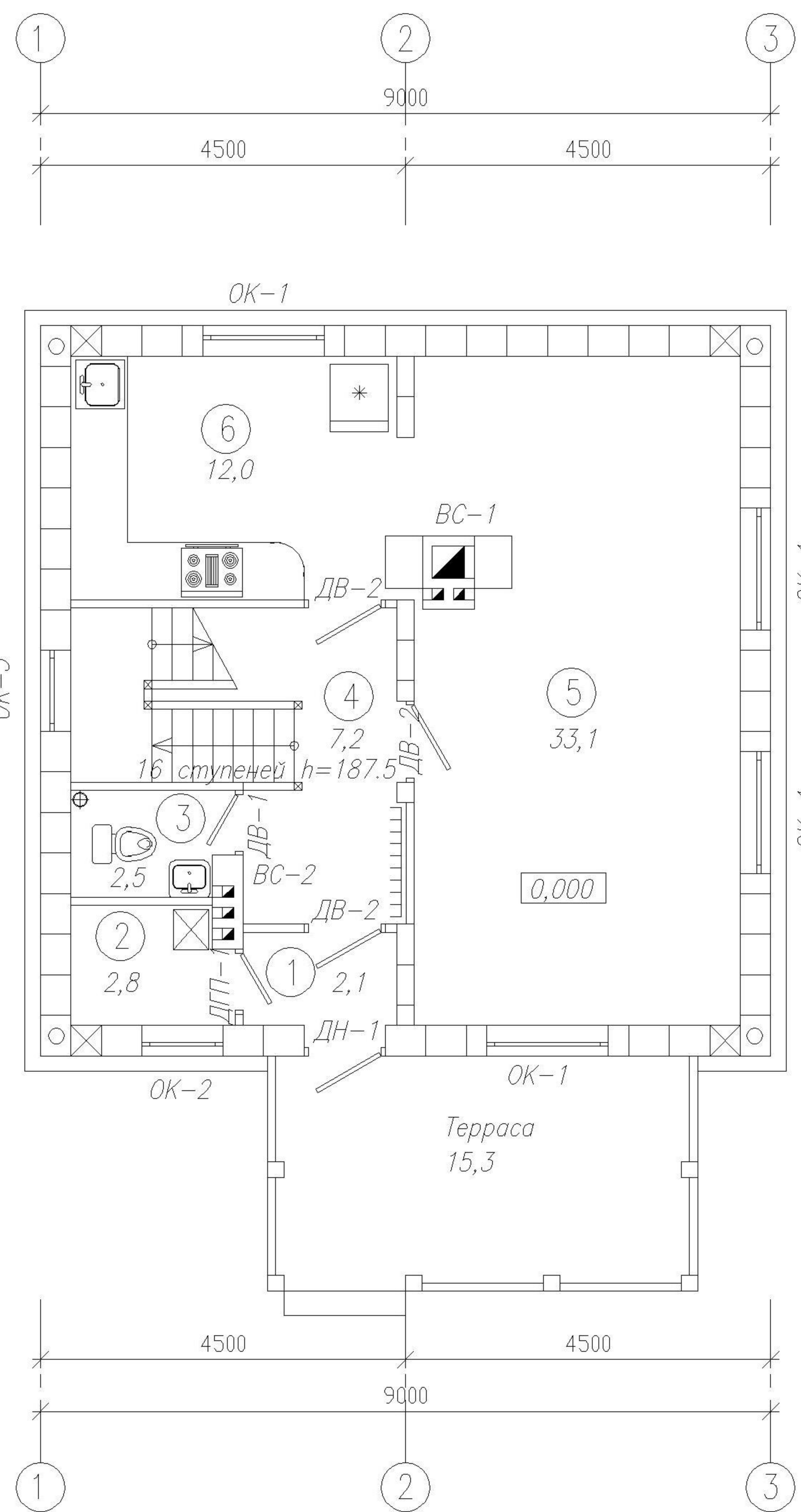
Экспликация 1-го этажа
