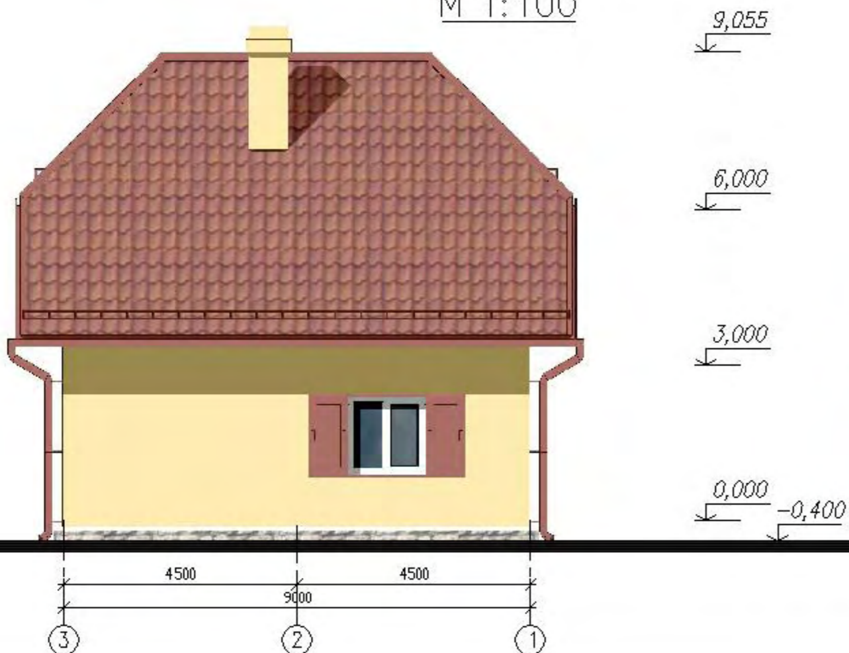
Фасад в осях 3-1 М 1:100
