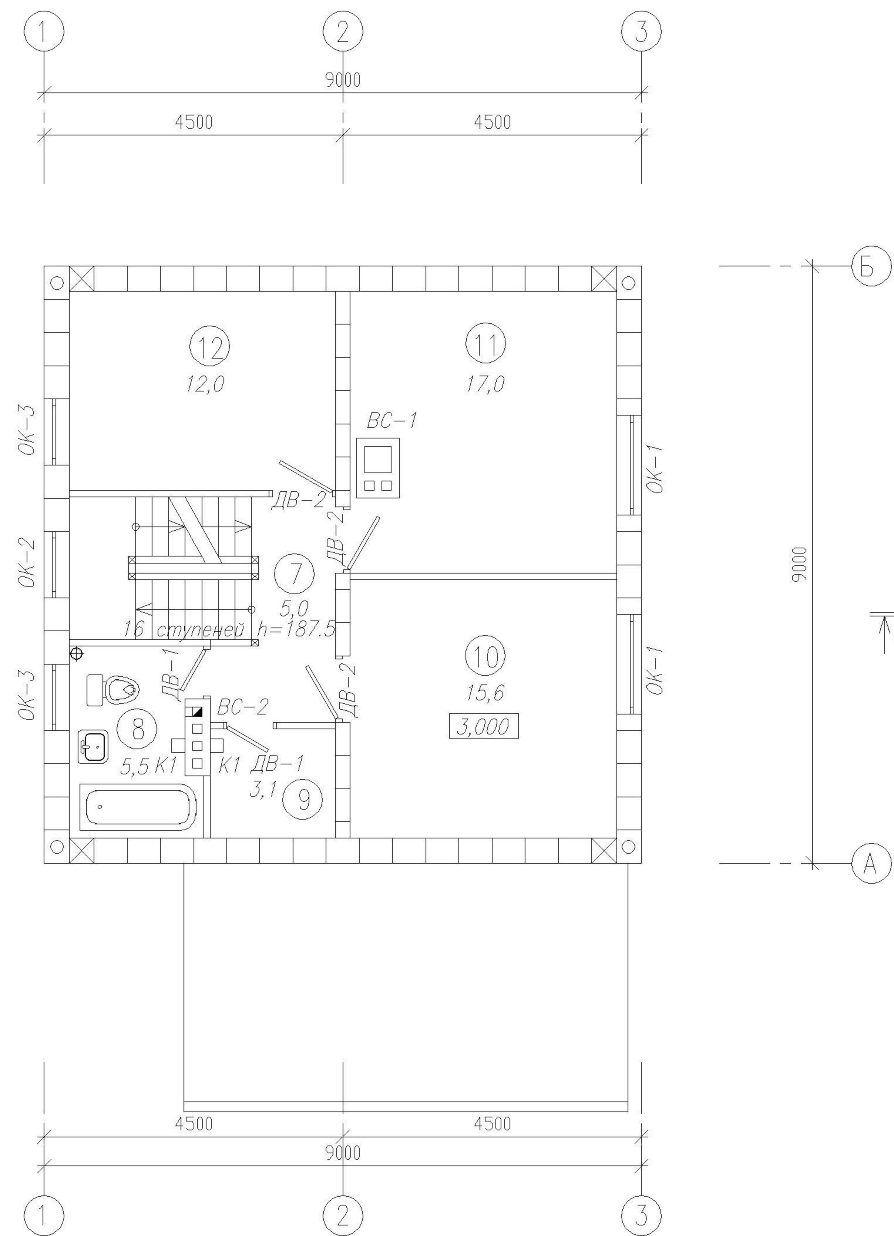
Экспликация 2-го этажа
